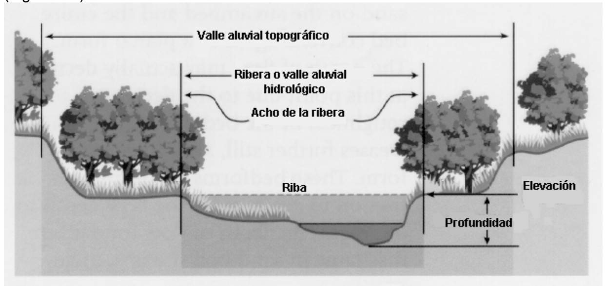
Figura 1.2 Componentes del valle aluvial y las orillas del arroyo.
