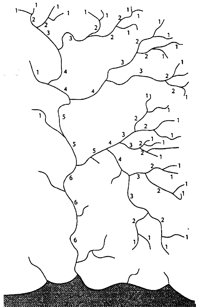
Figure 1.4 Orden del sistema de los ríos
