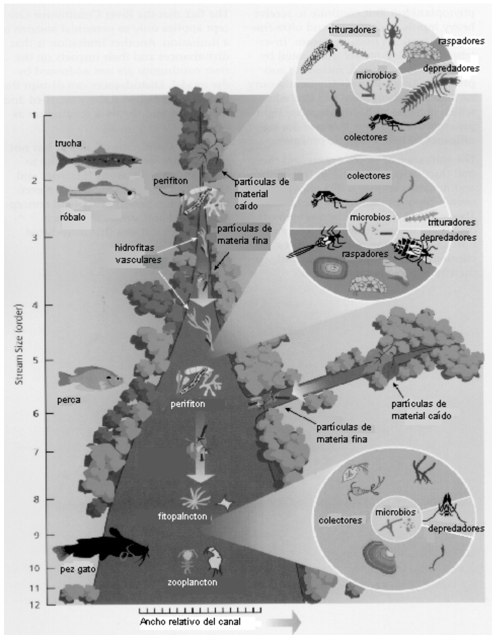
Figura 1.5 Modelo del Concepto de Continuum del Río
