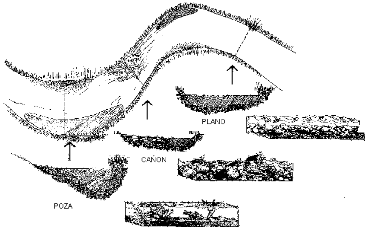
Figura 1.3. Componentes del Sistema de un Arroyo
